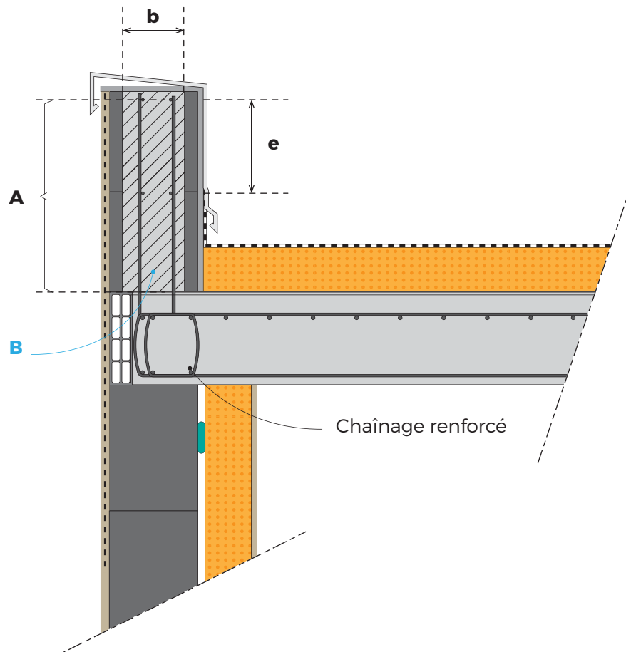
Figure 1 – Disposition concernant les acrotères bas NB: la section hachurée B à prendre en compte est celle du noyau de béton
